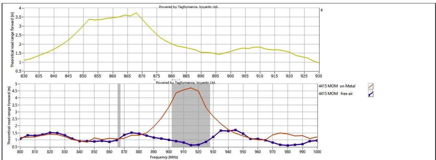
UNI 4415 - RF performance(M730)
